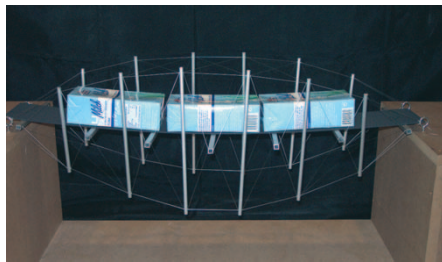
Belastungsversuch mit 3 Kg
