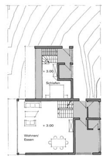
Ebene +3.00
