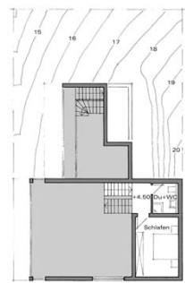
Ebene +4.50
