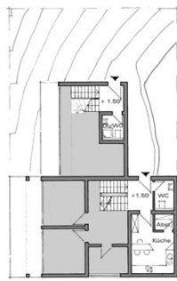
Ebene +1.50
