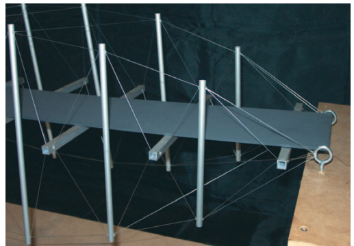
Tensegrity-Brücke _ Übung
