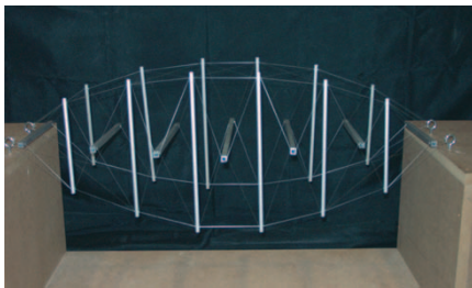
Brückentragwerk als Tensegrity-Konstruktion
